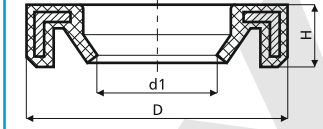
Teknik Çizim Drawing 2
