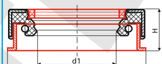
Teknik Çizim Drawing 6
