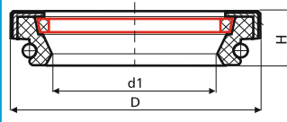
Teknik Çizim Drawing 23
