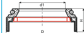
Teknik Çizim Drawing 14
