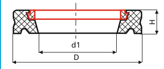
Teknik Çizim Drawing 27
