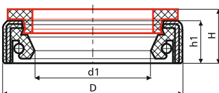
Teknik Çizim Drawing 20
