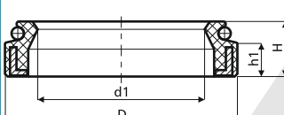
Teknik Çizim Drawing 8
