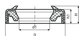
Teknik Çizim Drawing 29
