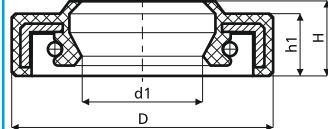
Teknik Çizim Drawing 1
