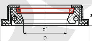
Teknik Çizim Drawing 25
