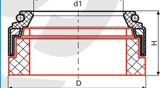
Teknik Çizim Drawing 19
