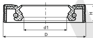
Teknik Çizim Drawing 18
