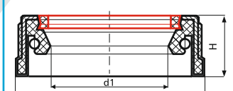
Teknik Çizim Drawing 13
