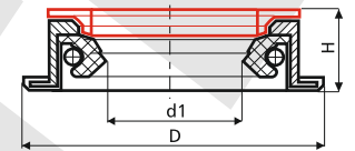
Teknik Çizim Drawing 22
