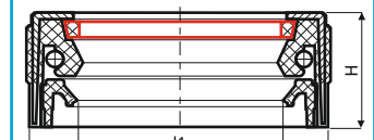
Teknik Çizim Drawing 15
