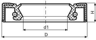
Teknik Çizim Drawing 16
