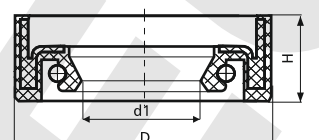
Teknik Çizim Drawing 28
