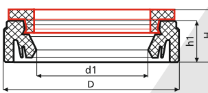
Teknik Çizim Drawing 21
