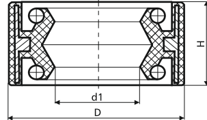
Teknik Çizim Drawing 17
