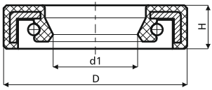
Teknik Çizim Drawing 0
