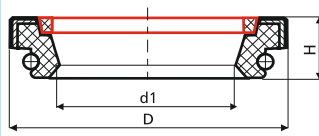
Teknik Çizim Drawing 26
