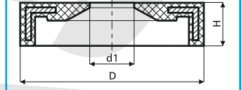
Teknik Çizim Drawing 3
