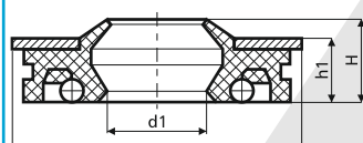
Teknik Çizim Drawing 5
