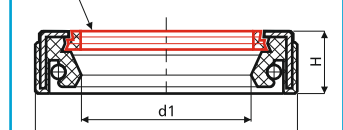
Teknik Çizim Drawing 11
